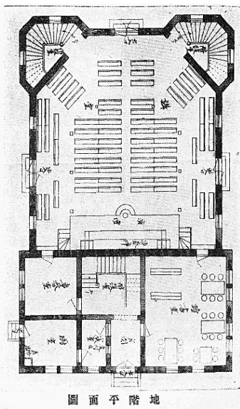
図3 青年仏教伝道会会堂設計図(『青年伝道』45号、1907年4月)
