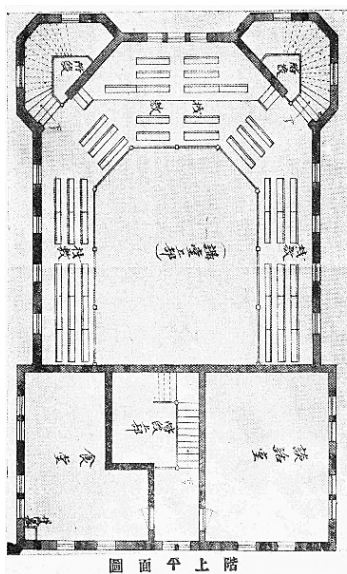
図3 青年仏教伝道会会堂設計図(『青年伝道』45号、1907年4月)
